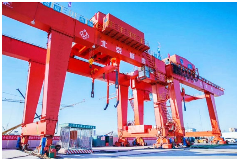
MGD 型盾构门式起重机 MGD shield gantry crane
