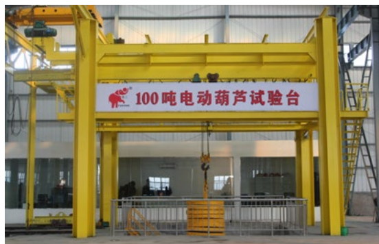
电动葫芦试验台 Electric hoist test platform
